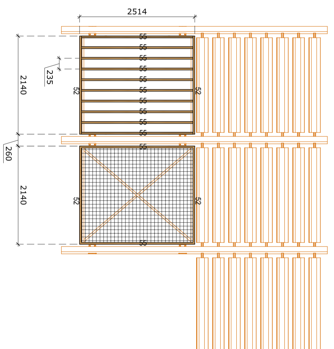
PARTICOLARE 4 - Dettaglio architrave portale e collegamento doghe scala 1:5 (misure in millimetri)
